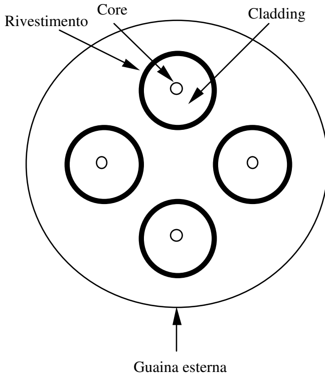
Figura 2-4: Sezione di un cavo contenente fibre ottiche
